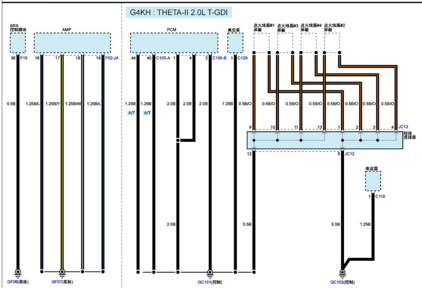
搭铁分布(13)
